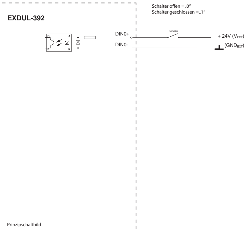
Graphik 14.1 Beschaltung des Optokopplereingangs
